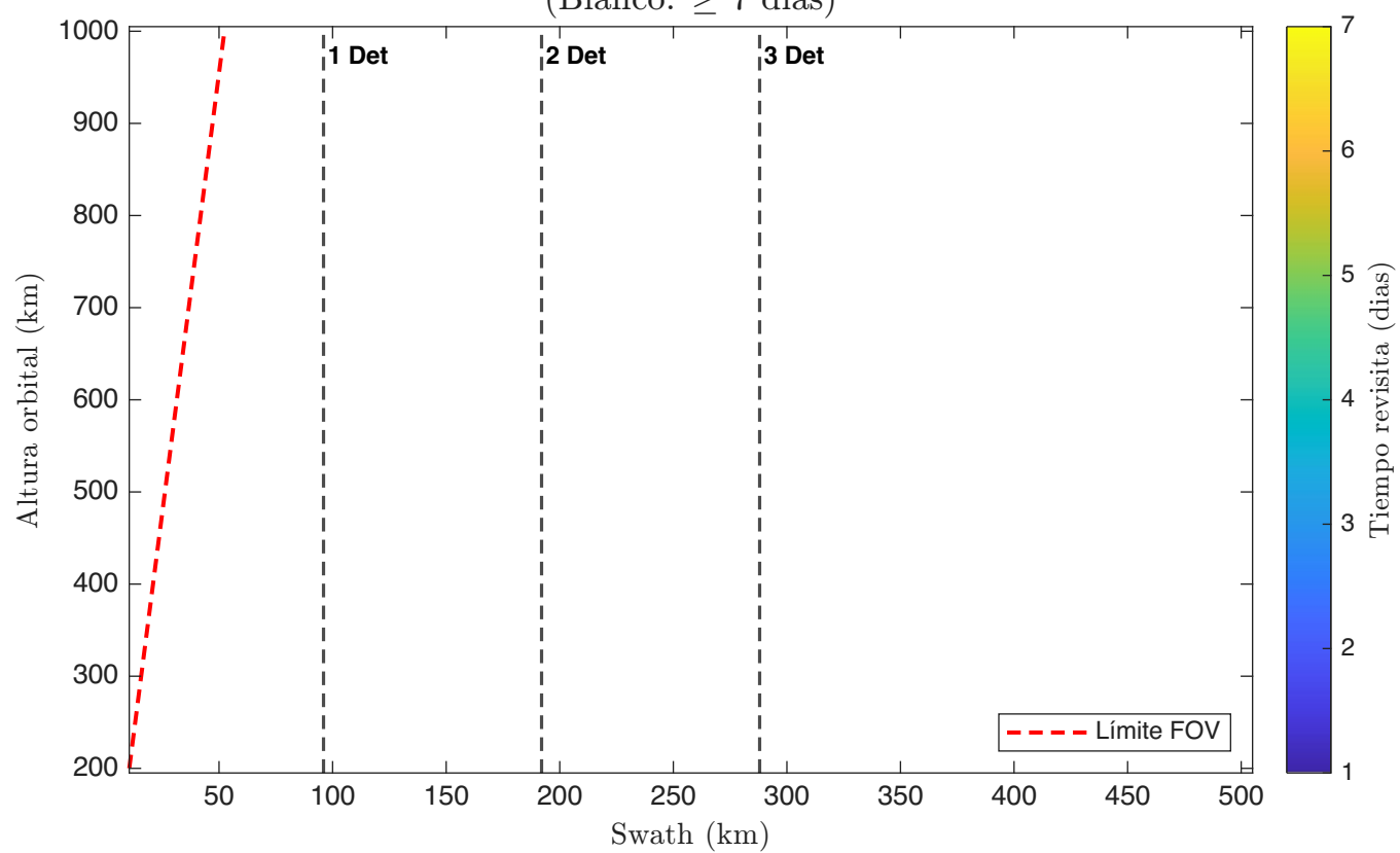
Tiempo Revisita - 2 Satellite(s); 1 Telescopio(s): Korsch; Detector 1 (Blanco: \geq 7 dias)
